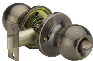
ЗАЩЕЛКА ВРЕЗНАЯ ЗЩ-607-ВК-АВ ФИКСАТОР ШАР БУЛАТ
